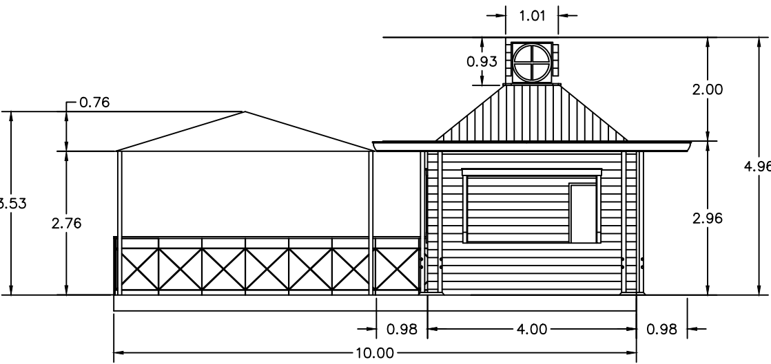
PROSPETTO POSTERIORE
