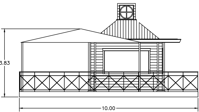
PROSPETTO FRONTE
