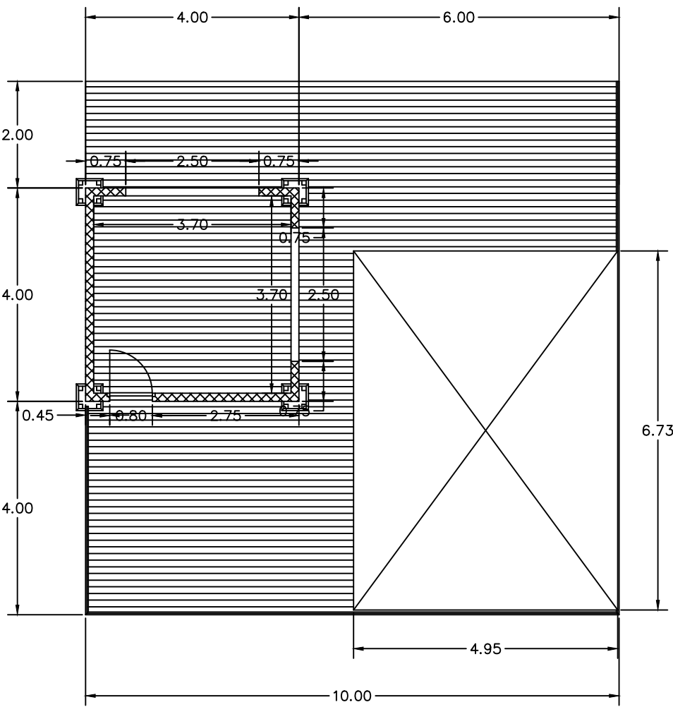
PIANTA QUOTATA
