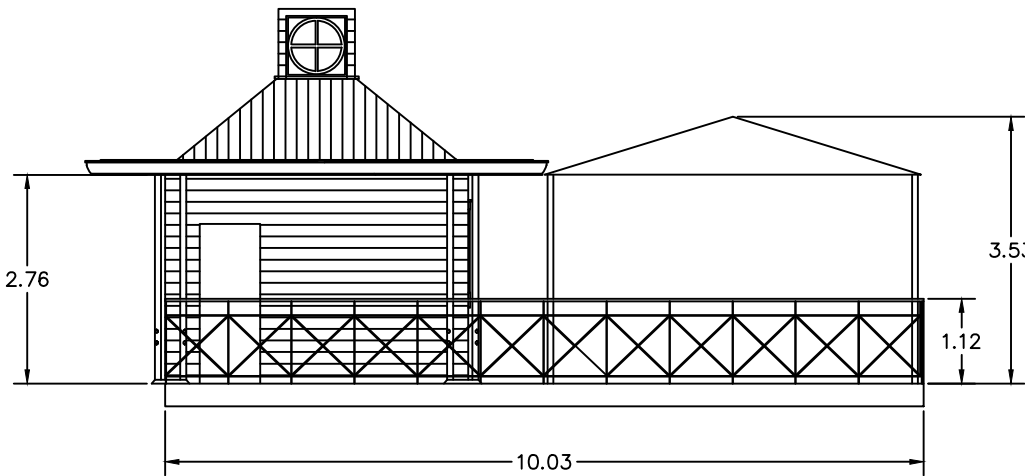
PROSPETTO POSTERIORE
