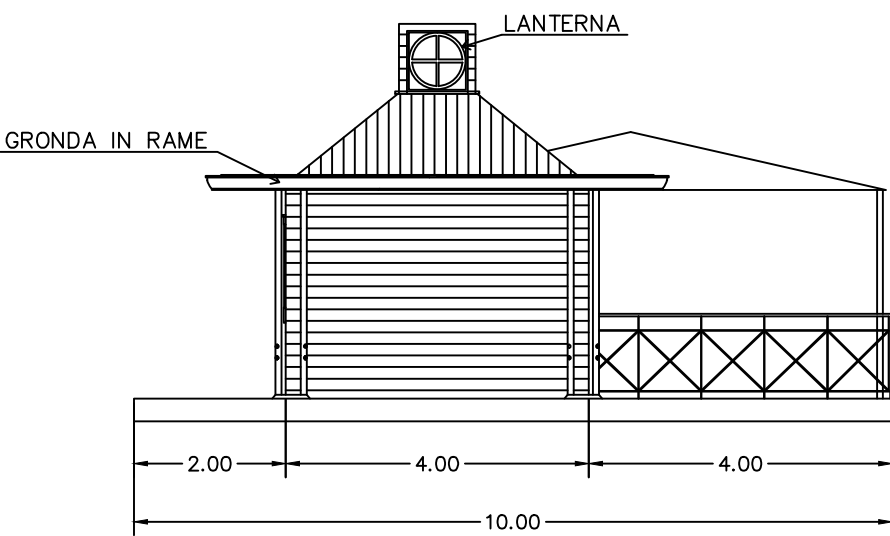
PROSPETTO LATERALE
