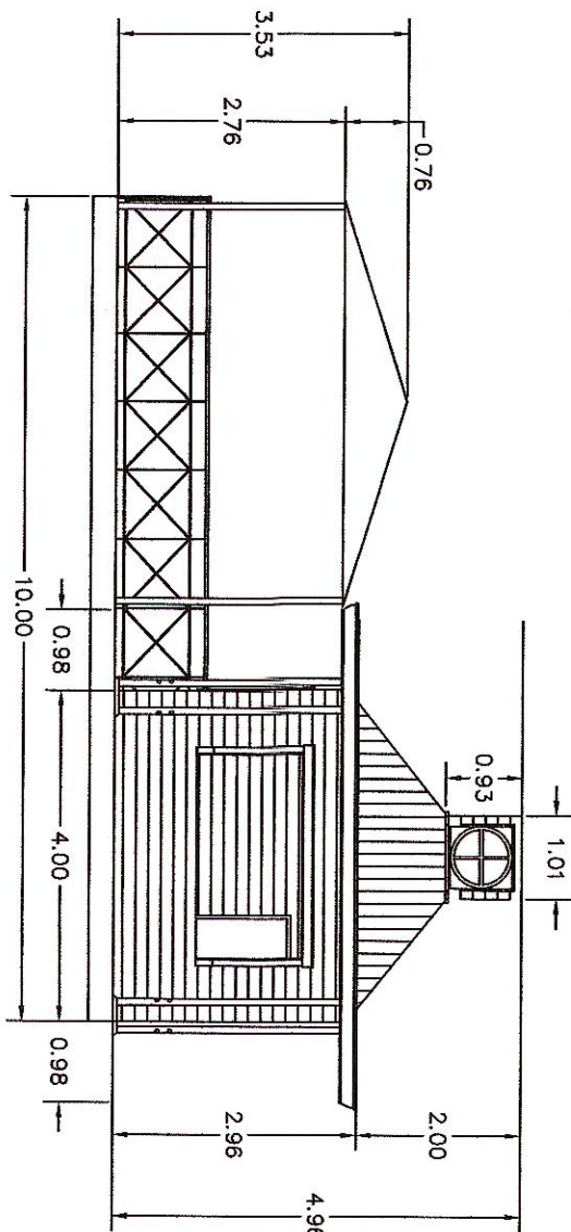
PROSPETTO FRONTE
