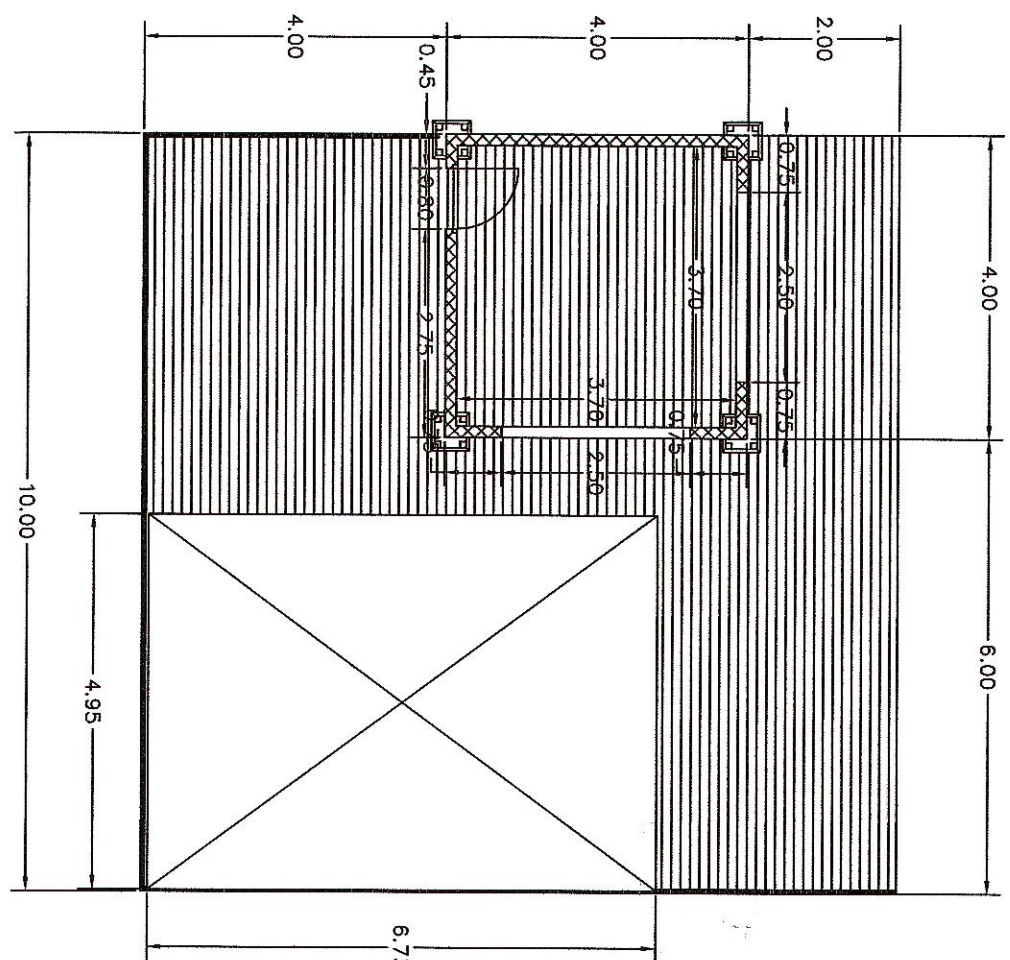
PIANTA QUOTATA
