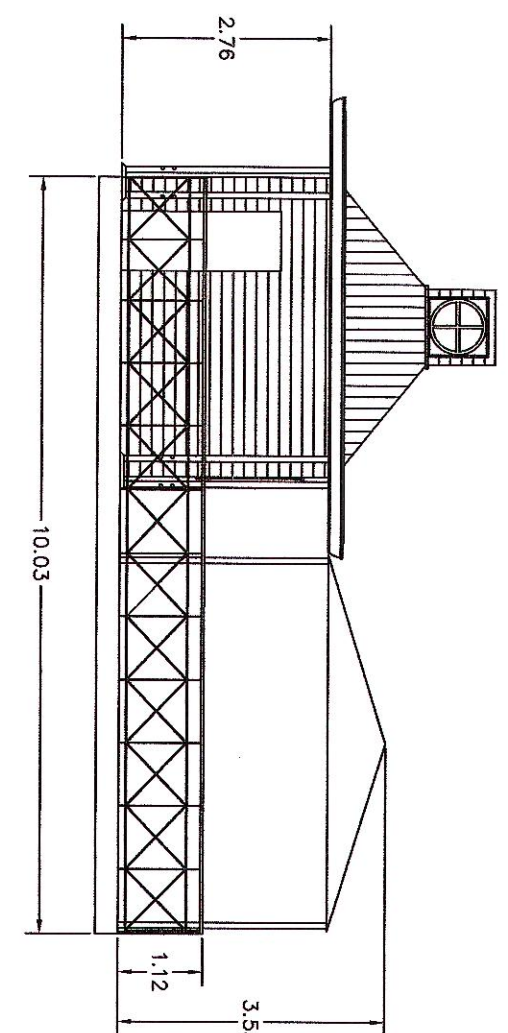
PROSPETTO POSTERIORE
